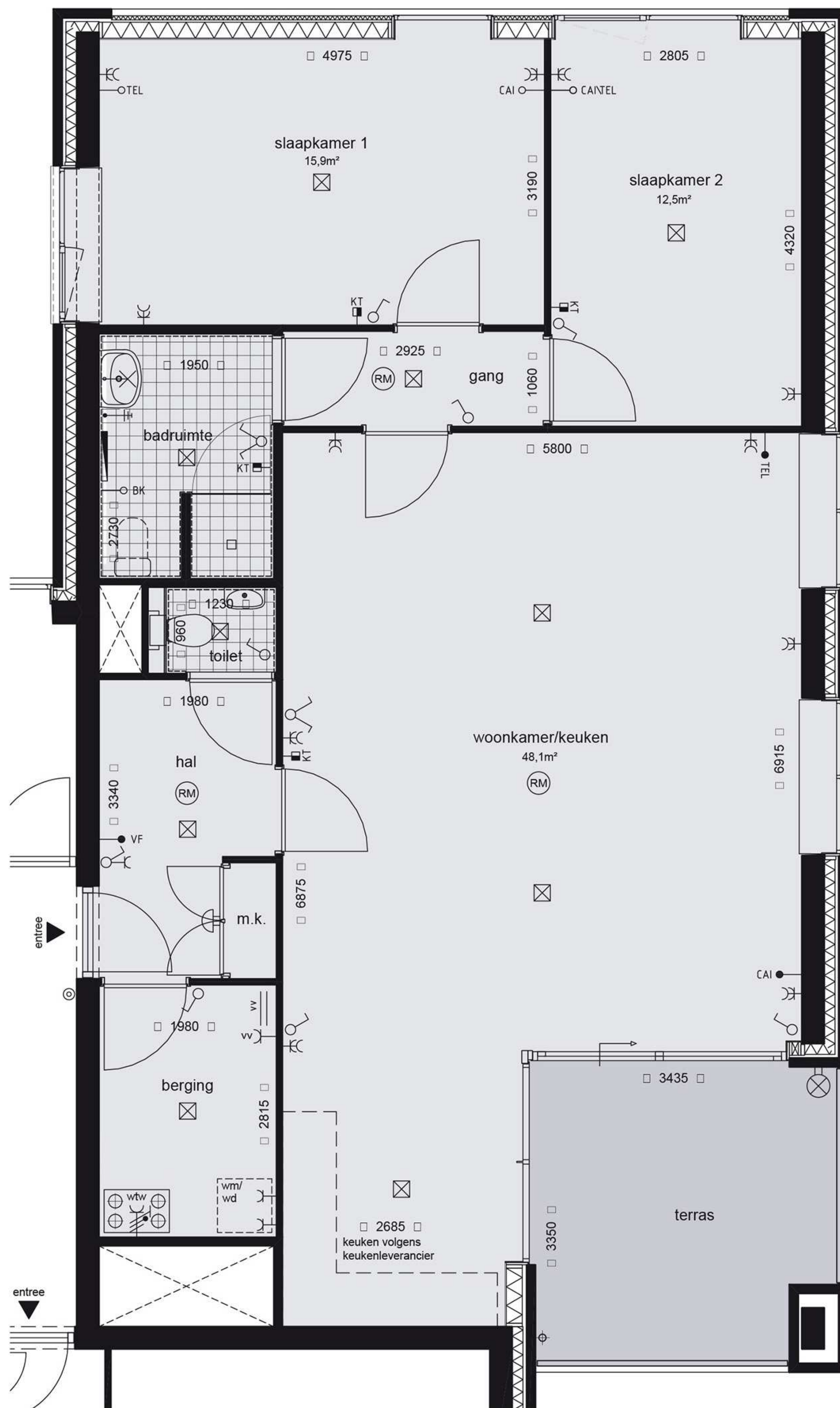
Getekende plattegrond, bouwnummers 34, 38, 42, 46 en 50
