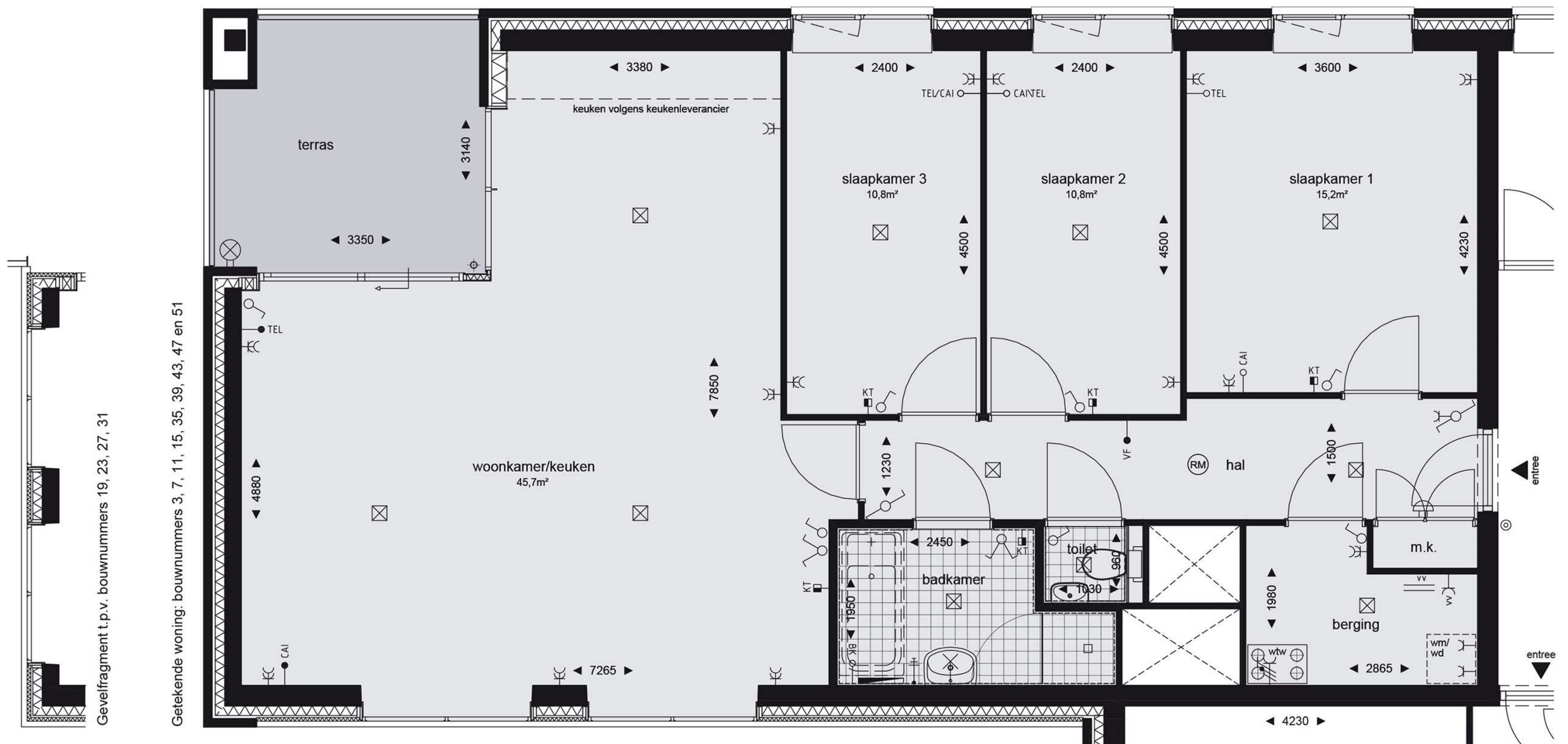
Getekende woning: bouwnummers 3, 7, 11, 15, 35, 39, 43, 47 en 51
